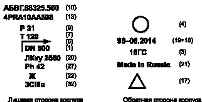
Рисунок Г.3 — Пример расположения маркировки на корпусе углового регулирующего клапана
