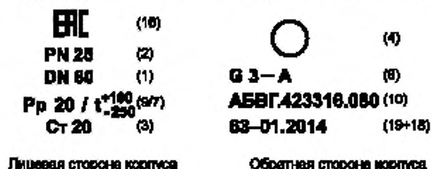
Рисунок Г.1 — Пример расположения маркировки на корпусе запорной арматуры
