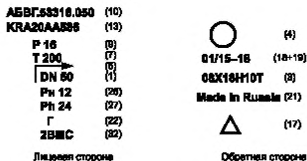
Рисунок Г.2 — Пример расположения маркировки на корпусе предохранительного клапана
