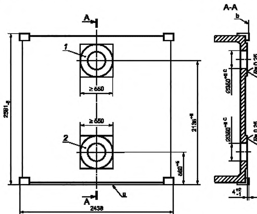
Рисунок В.1 — Размеры отверстий для воздуха в торцевых стенках изотермических контейнеров типа 1AA
