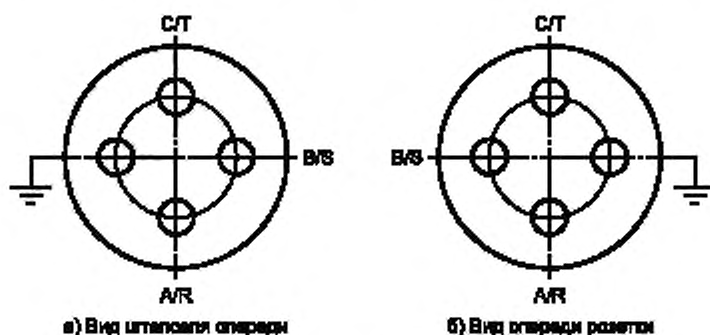
Рисунок Г.1 — Штепсель и розетка (вид спереди)
