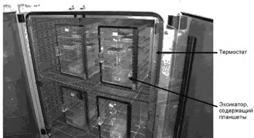
Рисунок 4 — Устройство для инкубации личинок
