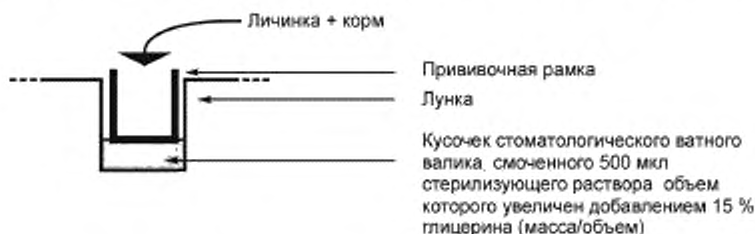
Рисунок 1 — Рамка с личинками в лунке с культурой ткани
