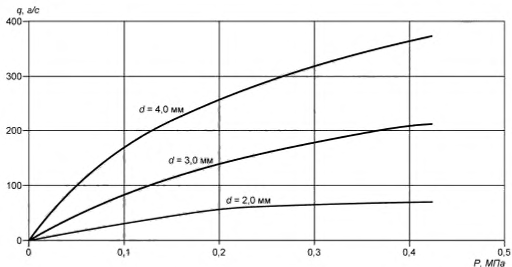
Рисунок 1 — Пример тарифовочных кривых расхода удобрения через распылители (жиклеры)
