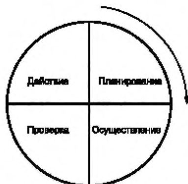
Рисунок 1 — Цикл Шухарта–Деминга
