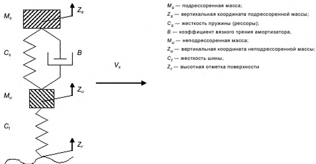
Рисунок В.1 — Модель автомобиля для расчета IRI
