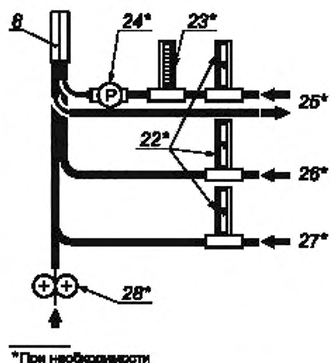
Рисунок А.6 — Блок питания
