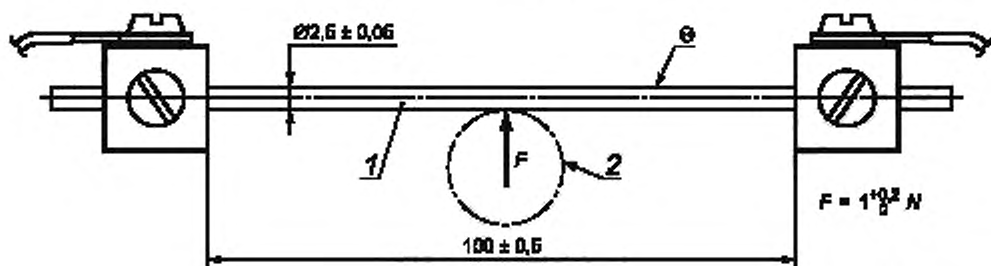
Рисунок 1 — Устройство для проверки стойкости изоляции к воздействию горячих предметов
