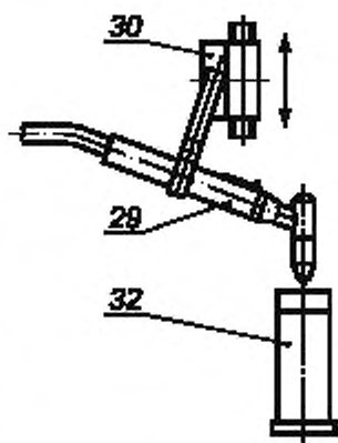
Рисунок В.3 — Горелки для плазменной сварки
