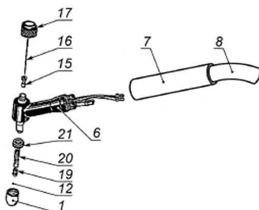
Рисунок А.4 — Горелка для плазменной сварки
