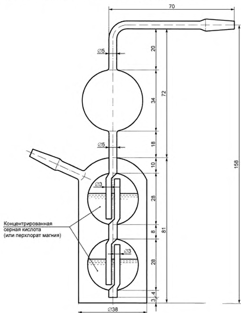
Рисунок 2 — Блок абсорбции
