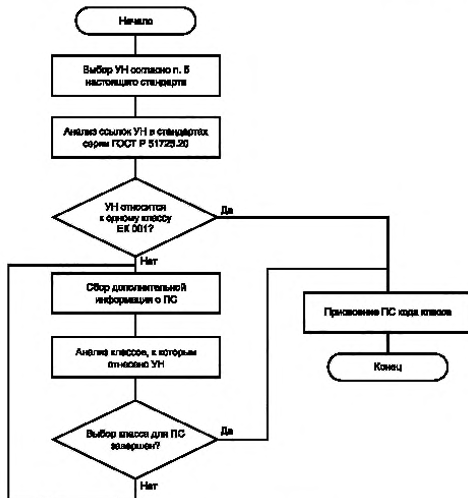
Рисунок 2 — Алгоритм классификации ПС
