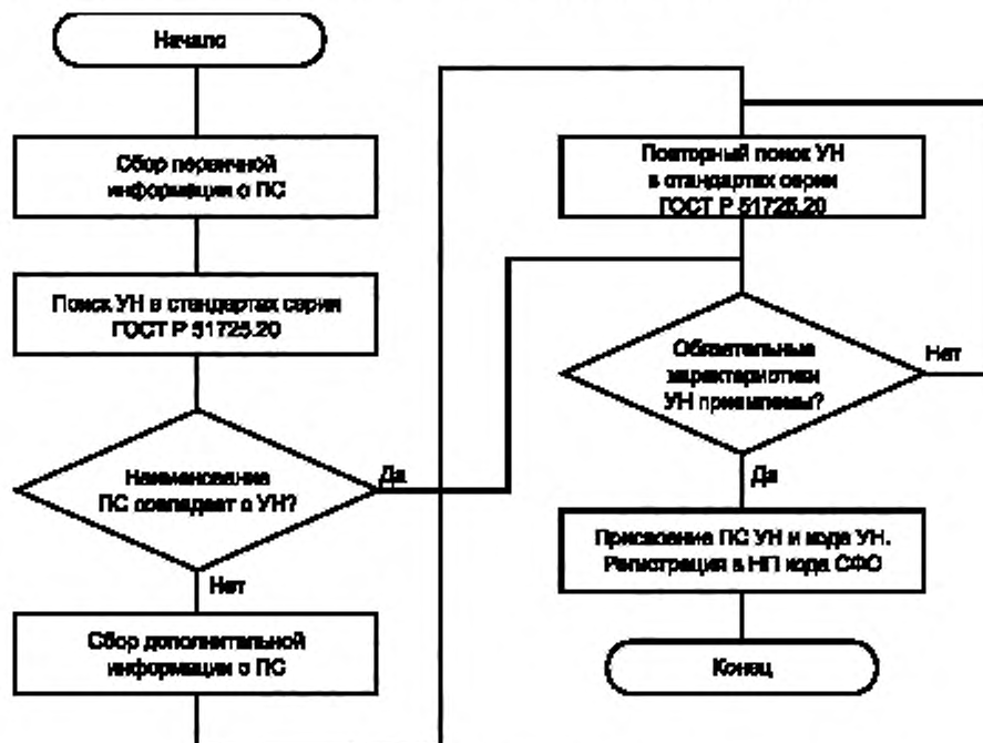
Рисунок 1 — Алгоритм идентификации ПС для описания в ФКП
