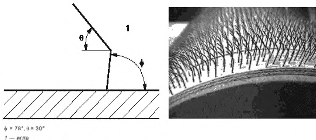
Рисунок 1 — Электромеханический разрыхлитель
