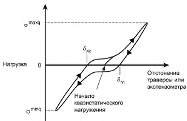
Рисунок 2 — Параметры петли гистерезиса для расчета смещения крепежа в зависимости от количества циклов нагружения
