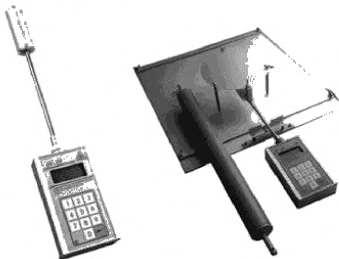
Рисунок 1 — Прибор для измерения напряженности электростатического поля СТ-01
