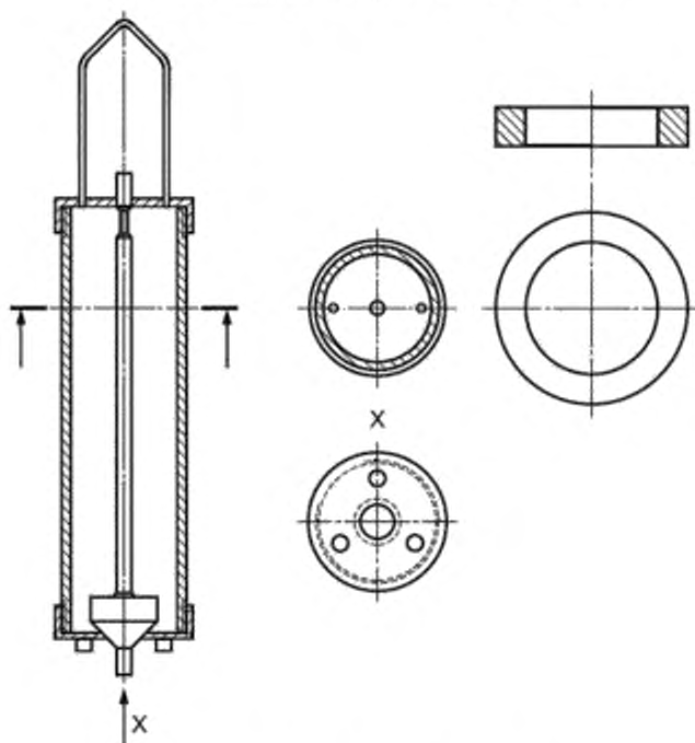
б) С клапаном собственного веса
