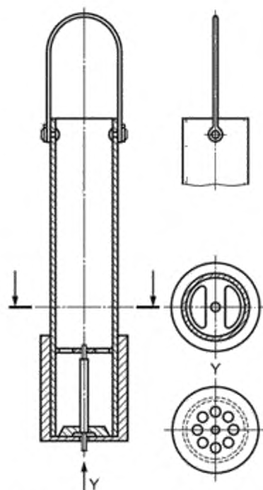
Рисунок А.9 – Пробоотборный цилиндр с клапаном (пробоотборник-грузило)
