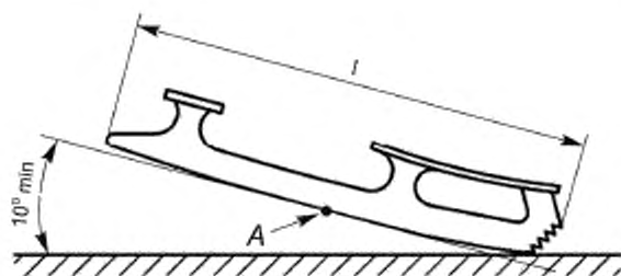
А — точка, через которую проводят касательную для измерения угла ( A = 1/2l ); l — длина полоза конька
