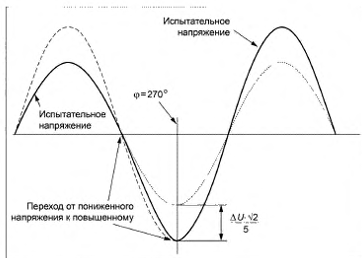
Рисунок 1с — Пример шага напряжения при возрастающем напряжении
