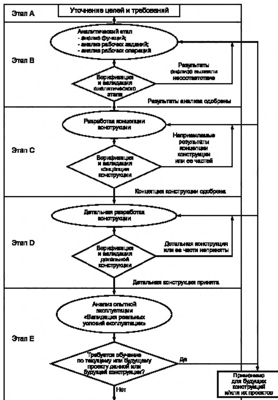
Рисунок 2 — Верификация и валидация при проектировании
