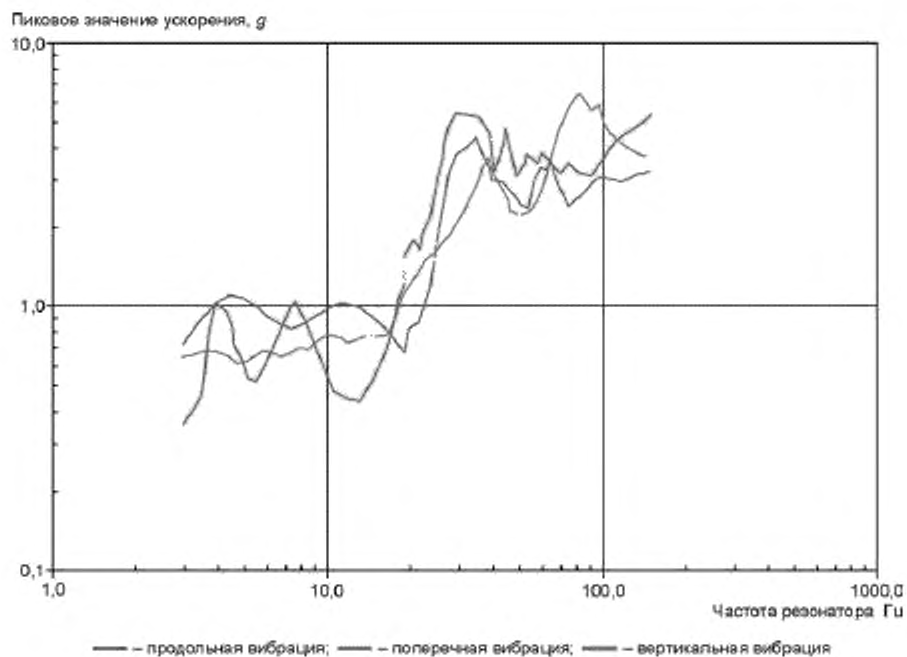
Рисунок 30 — Ударные спектры для повторяющихся событий, по данным [11] ( \zeta = 3\% , Q = 16,6 )
