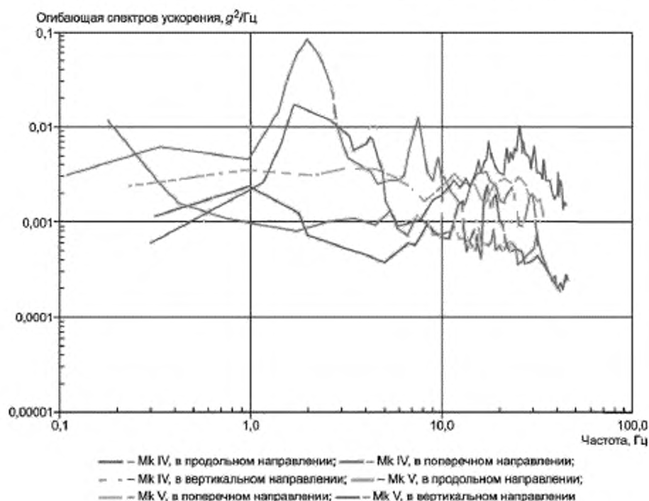
Рисунок 24 — Огибающие спектров ускорения на ролдрейлерах (Американские железные дороги)
