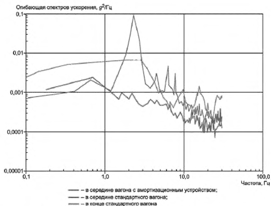
Рисунок 18 — Огибающие спектров для вибрации товарных вагонов в поперечном направлении (Американские железные дороги)
