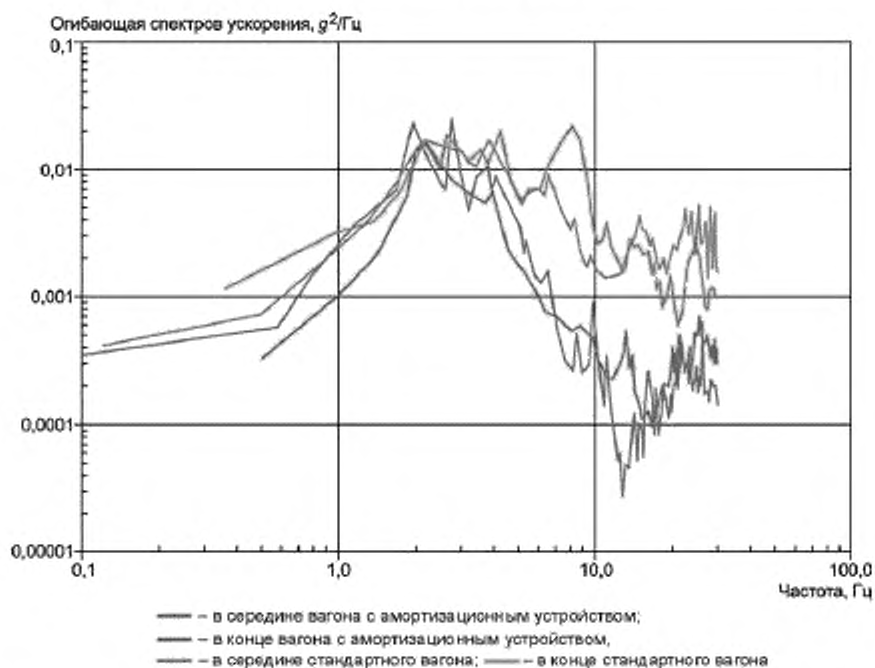
Рисунок 17 — Огибающие спектры для вибрации товарных вагонов в вертикальном направлении (Американские железные дороги)
