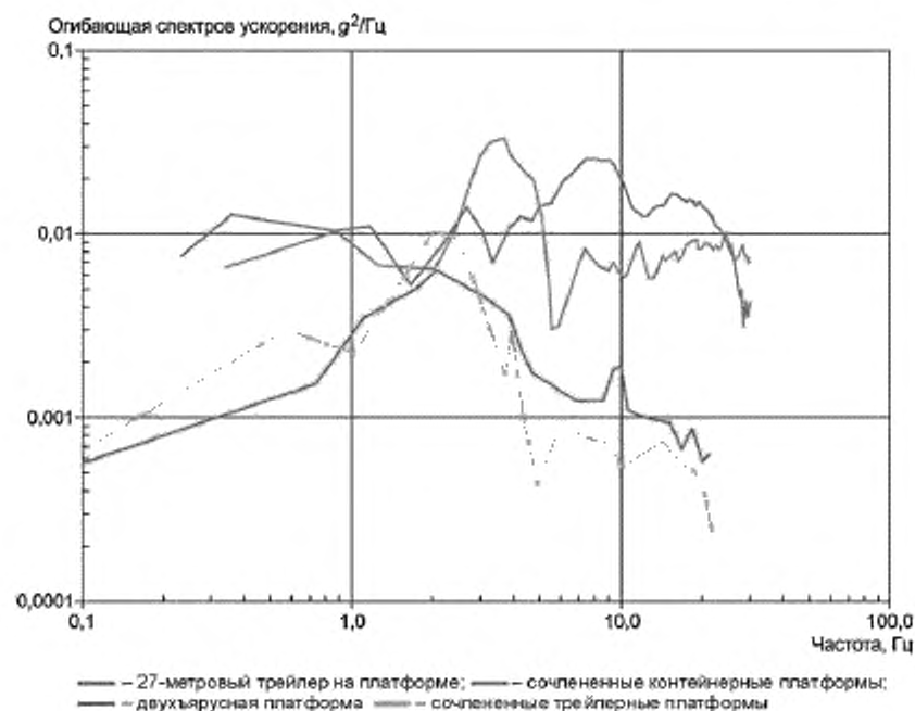
Рисунок 16 — Огибающие спектры для вибрации в продольном направлении при смешанных перевозках (Американские железные дороги)
