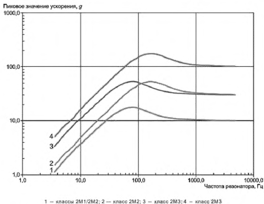
Рисунок 42 — Тестовые воздействия МЭК 60721-3-2:1997 (ударные спектры)
