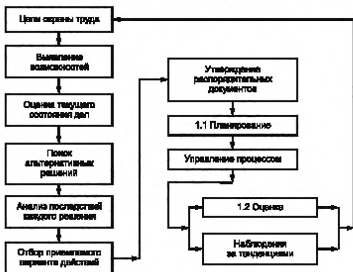
Рисунок 4 — Схема процесса управления производственной безопасностью в организации
