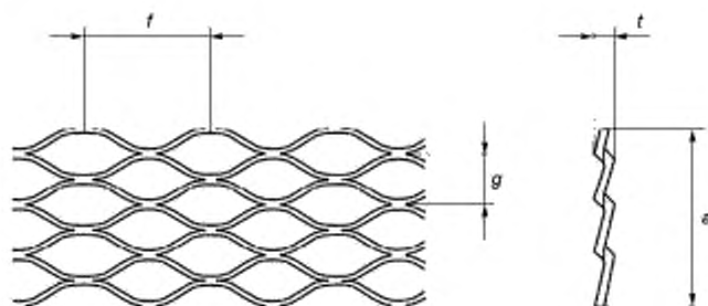
Рисунок 5.4 — Просечно-вытяжная сетка
