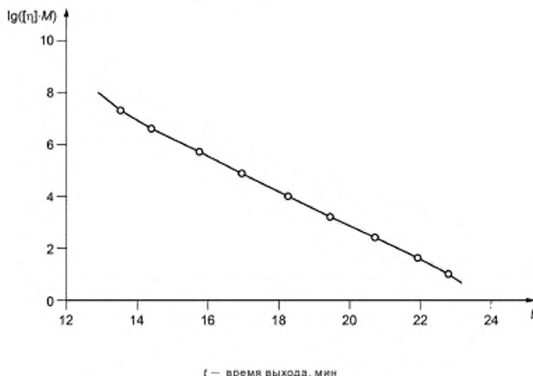
Рисунок 1 — Универсальная калибровочная кривая
