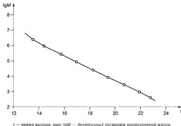
Рисунок 2 — Калибровочная кривая для образца полимера [молекулярная масса M полимера рассчитана по формуле (A.4) или (A.6)]
