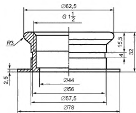
Рисунок А.2 — Горловина бочонка
