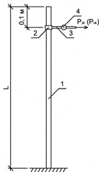
Рисунок А.1 — Схема испытания опоры на прочность и жесткость
