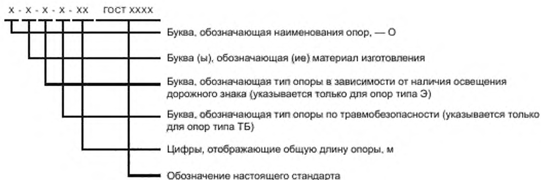
Рисунок 1 — Схема условного обозначения опор
