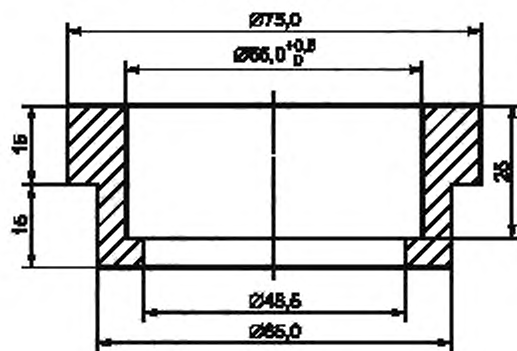
Рисунок 4 — Стопорное кольцо
