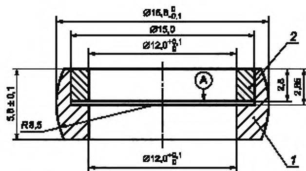
1 — держатель; 2 — стопорное кольцо
