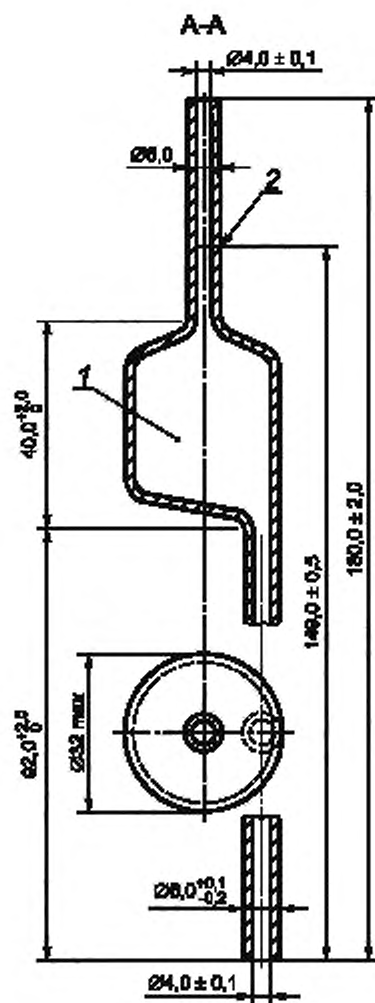
Рисунок 6 — Пипетка
