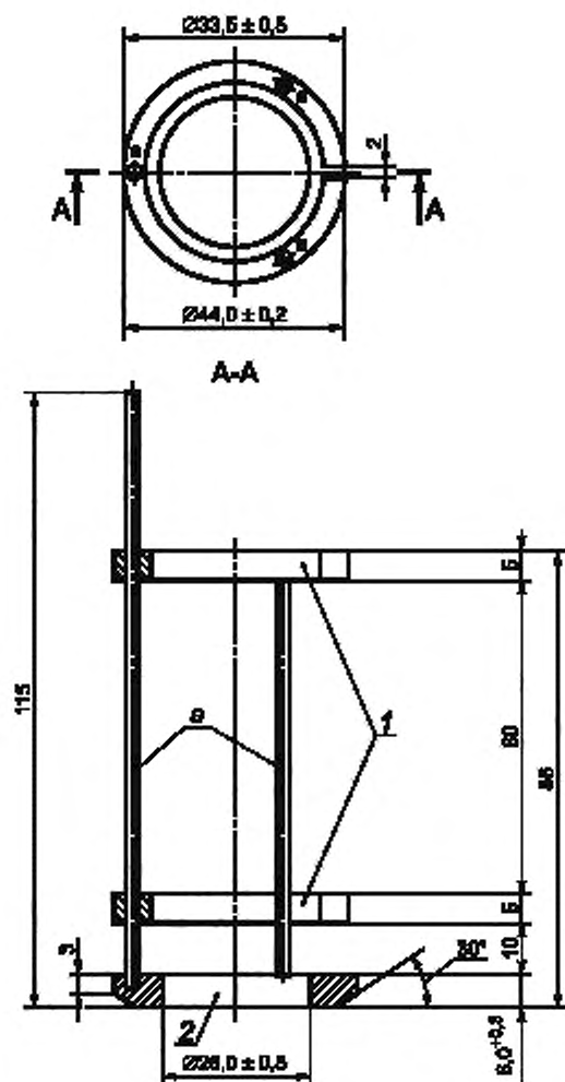
Рисунок 3 — Прокладки
