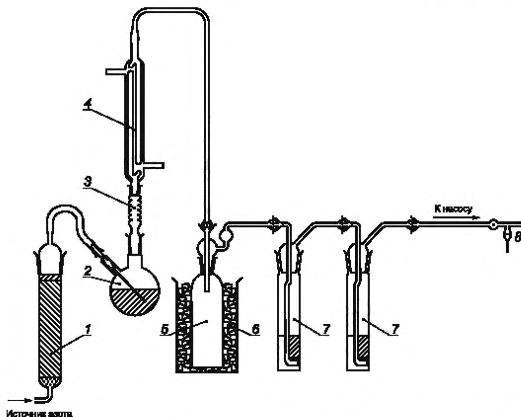
1 — поглотительная колба, заполненная раствором гашеной извести; 2 — круглодонная колба; 3 — перегонная колонка Вигре; 4 — холодильник с прямой трубкой; 5 — слянка для промывки газов; 6 — ледяная баня; 7 — поглотительные склянки; 8 — устройство управления всасывания
