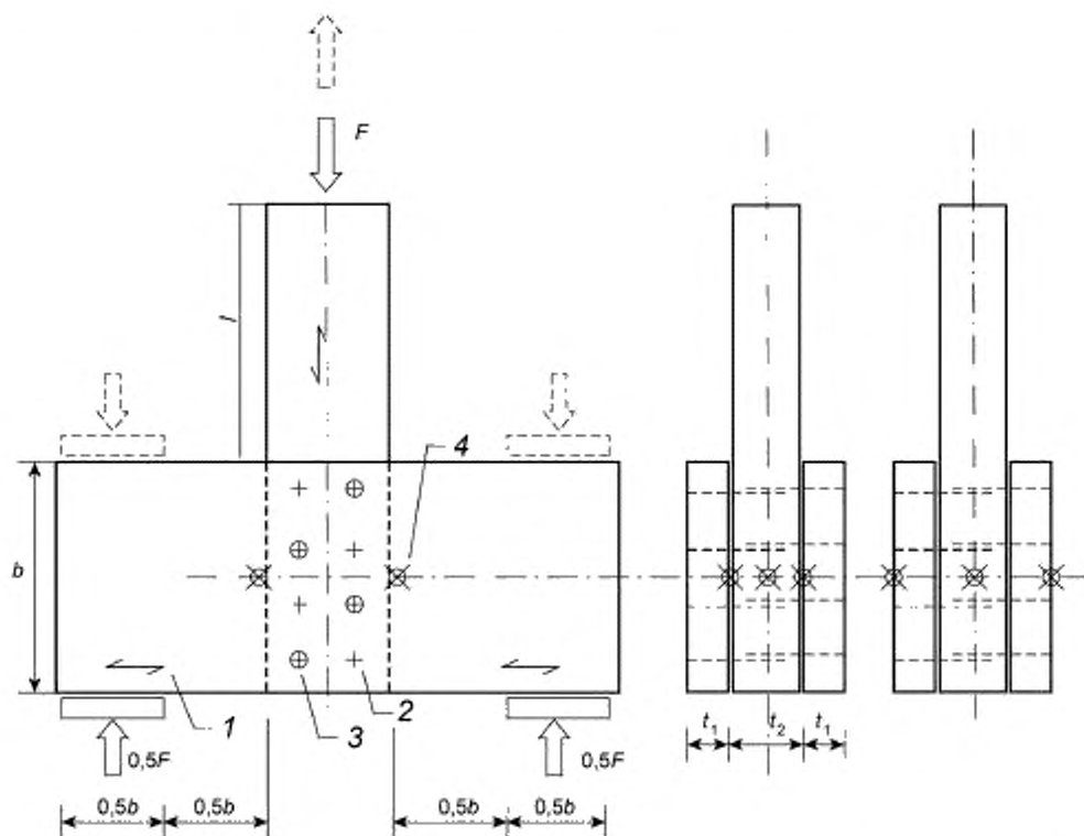
1 — направление волокон; 2 — невыступающая часть крепежа; 3 — выступающая часть крепежа; 4 — ⊕ точки измерения смещений; l — смещение элементов; t_1 — ширина крайнего элемента; t_2 — ширина среднего элемента
