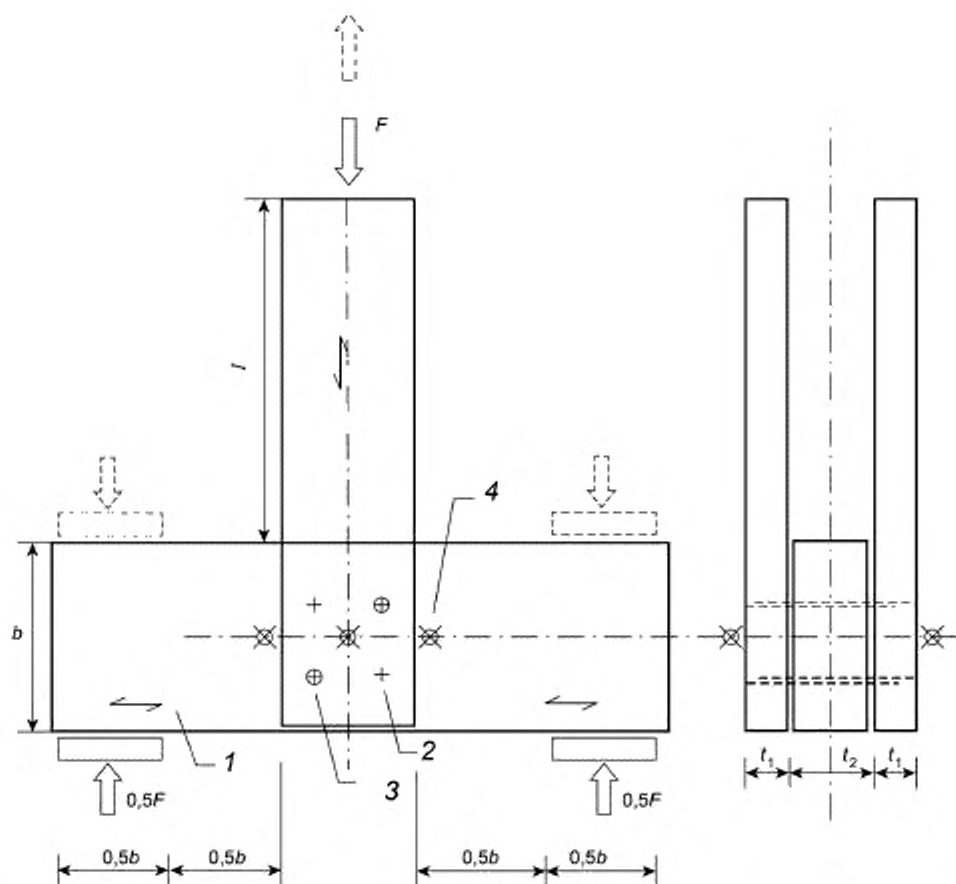
1 — направление волокон; 2 — невыступающая часть крепежа; 3 — выступающая часть крепежа; 4 — ⊕ точки измерения перемещений; l — величина смещения элементов; t_1 — ширина крайнего элемента; t_2 — ширина среднего элемента
