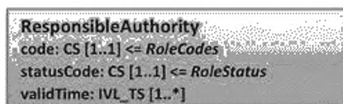
Рисунок 5 — Класс ResponsibleAuthority
