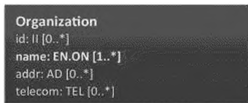
Рисунок 11 — Класс Organization
