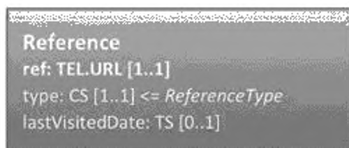
Рисунок 8 — Класс Reference
