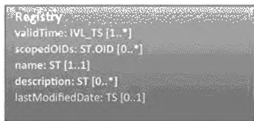
Рисунок 2 — Класс Registry
