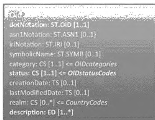
Рисунок 3 — Класс Oid
