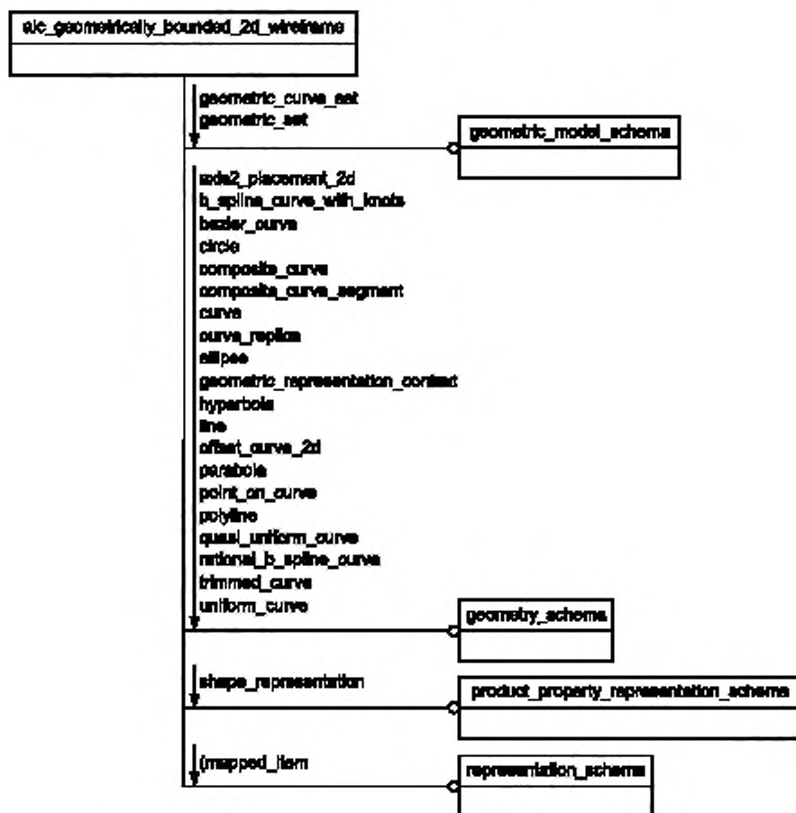
Рисунок D.1 — EXPRESS-G диаграмма схемы aic_geometrically_bounded_2d_wireframe. Диаграмма 1 из 2
