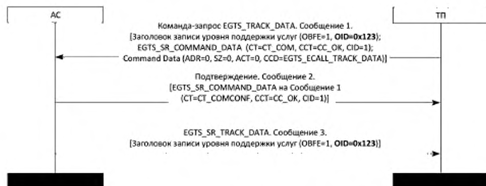
Рисунок 6 — Алгоритм способа использования OID
