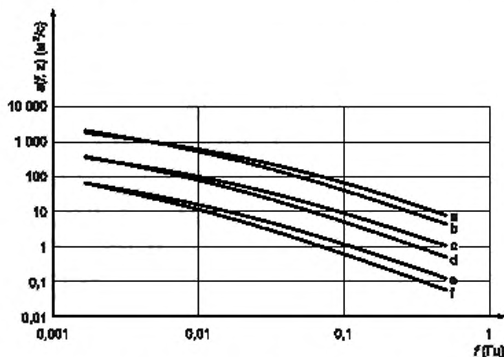
Рисунок А.1 — Примеры спектров (скорости) ветра
