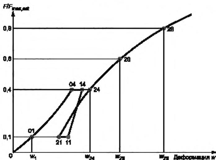
Рисунок 4 — Идеализированная кривая «нагрузка — деформация» и система измерений
