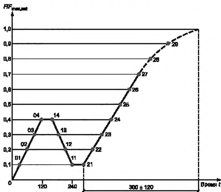
Рисунок 3 — Методика нагружения
