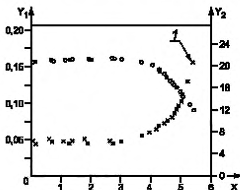
X — количество циклов N ( \times 10^4 ); Y_1 — потеря X ; Y_2 — модуль, ГН·м -2 ; 1 — точка разрушения Рисунок В.2 — Динамический модуль упругости и изменения затухания
