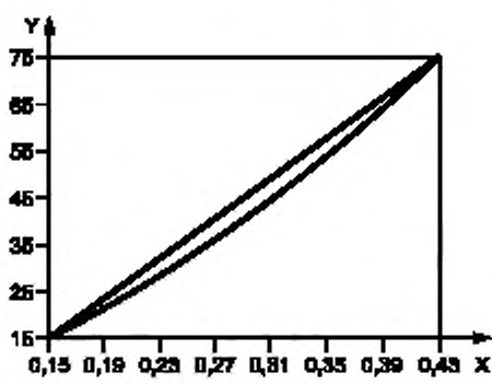
X — растяжение, %; Y — напряжение, МН·м -2 Рисунок В.1 — Типовая петля гистерезиса
