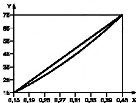
Рисунок А.1 — Типовая петля гистерезиса
