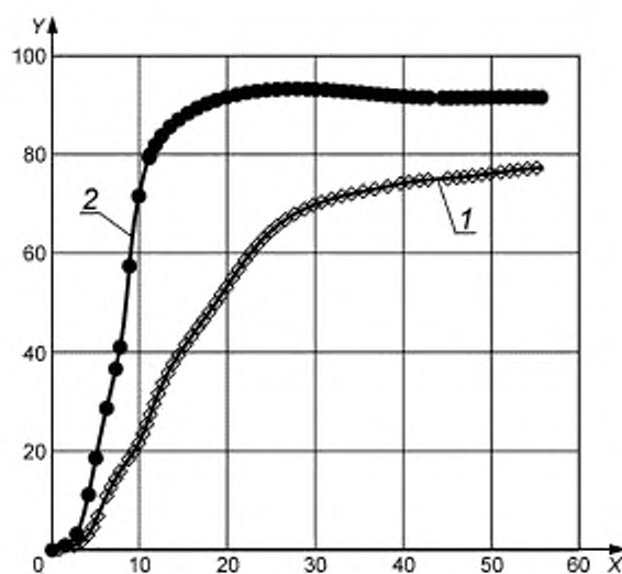
Рисунок А.6 — результаты испытания на биоразложение порошка ПКЛ [средний размер частиц — (180,7 \pm 76,8) мкм] в процессе контролируемого компостирования при 58^\circ\text{C} в соответствии с ГОСТ Р 57219. (в качестве контрольного материала использовали порошок целлюлозы с размером частиц менее 20 мкм)
