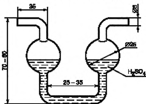
Рисунок 2 — Насадка
