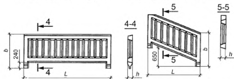
Панель ограждения платформы
