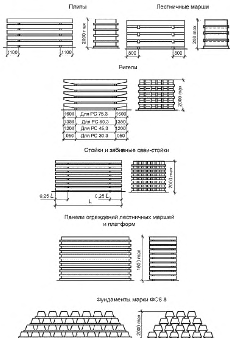
Рисунок А.1 — Схемы складирования
