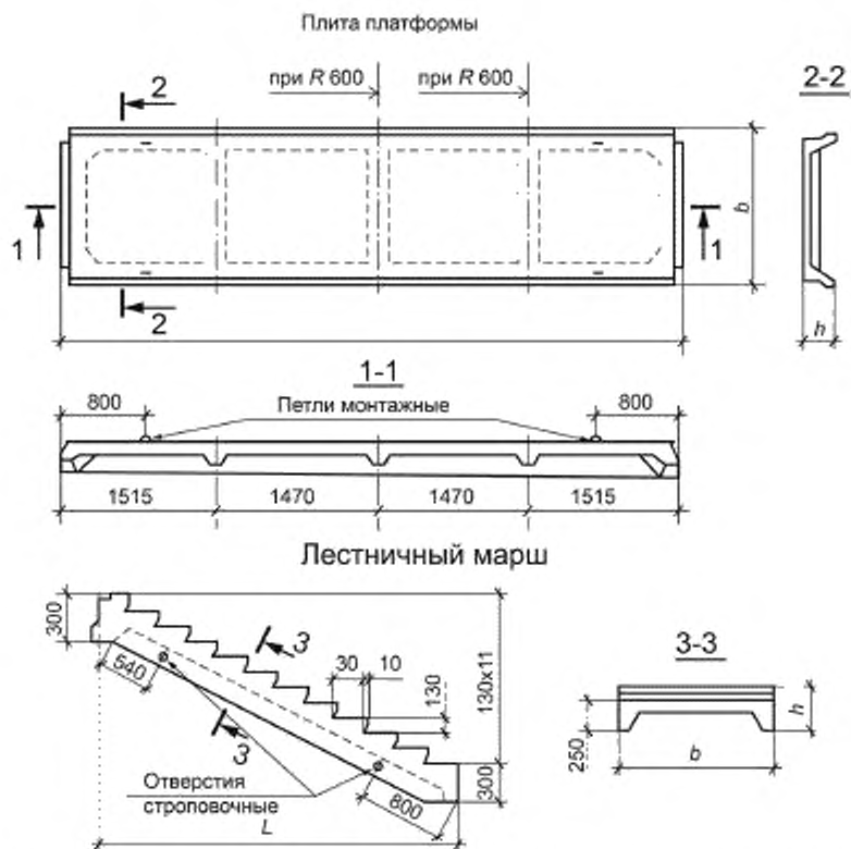
Рисунок 1 — Форма и размеры плит и лестничных маршей
