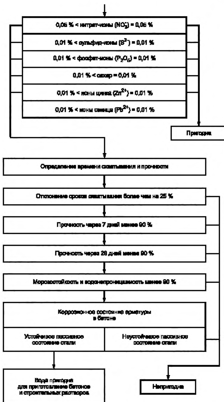
Рисунок Б.1, лист 2
