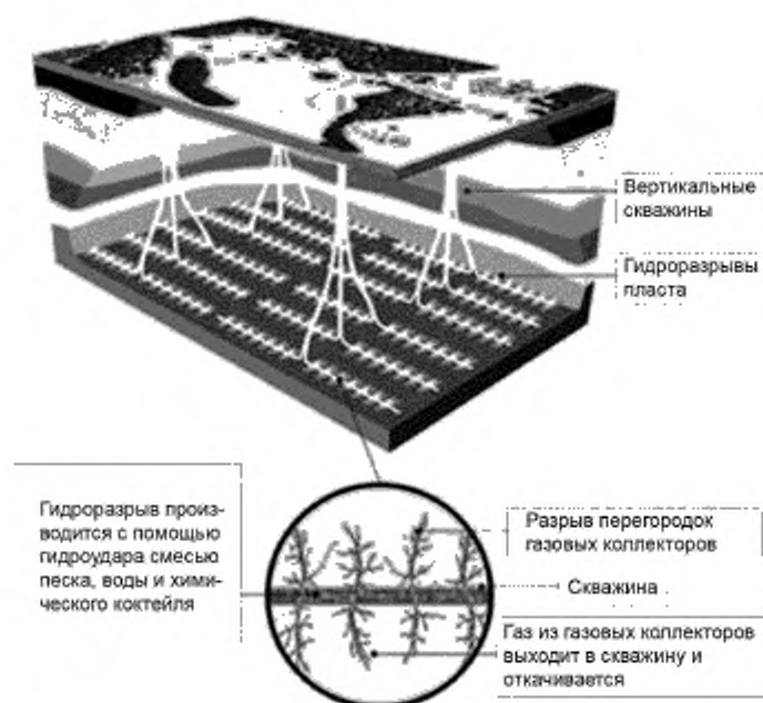
Рисунок 4 — Бурение одноствольных и многоствольных горизонтальных скважин с последующим использованием гидроразрыва пласта
