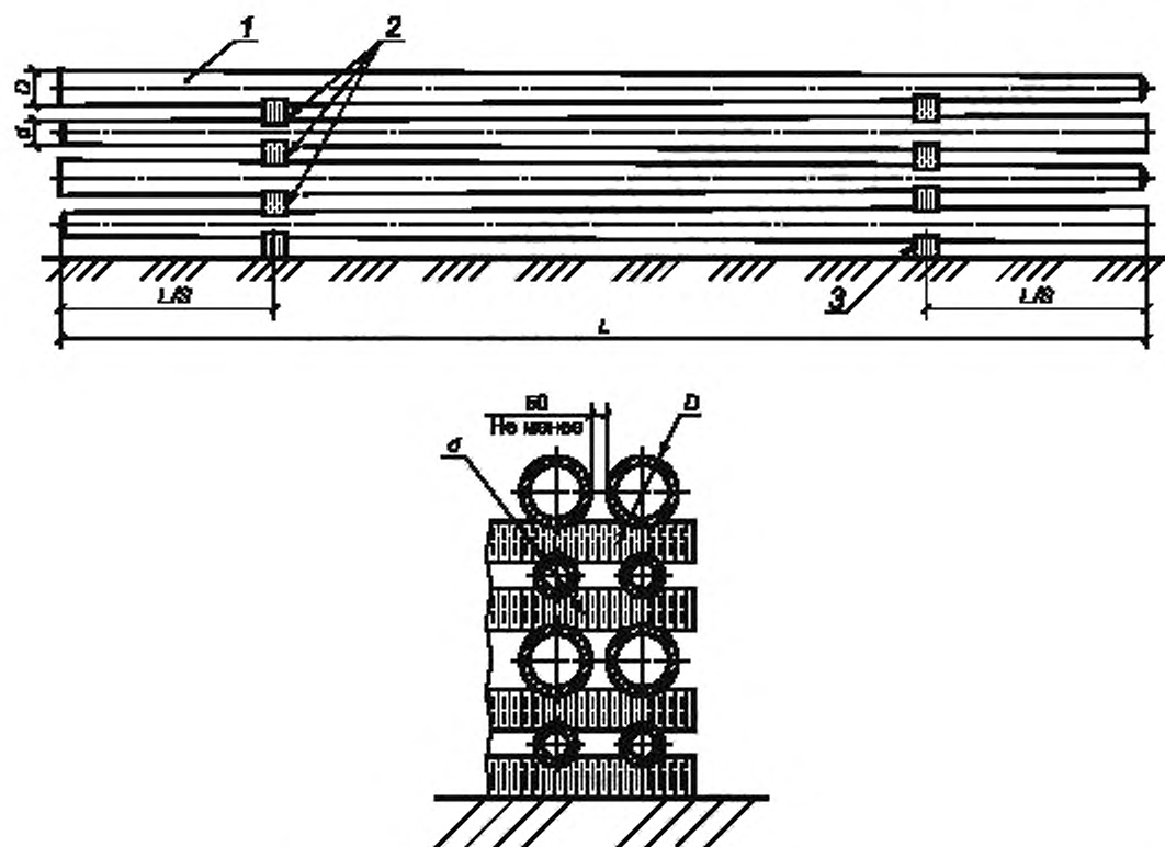
1 — стойка; 2 — прокладки, 3 — подкладка; L — длина стойки; D — диаметр нижней концы; d — диаметр верхней концы
