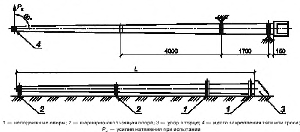
Рисунок 3 — Испытания стоек
