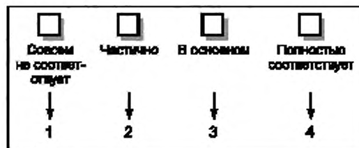
Рисунок 4 — Кодирование ответов
