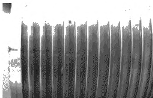
Рисунок 17 — Трещина на заходной фаске и наружной резьбе
