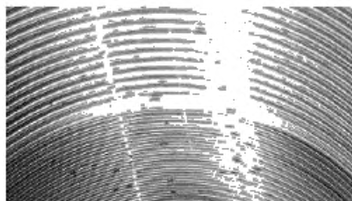
в) Следы коррозии на внутренней резьбе
