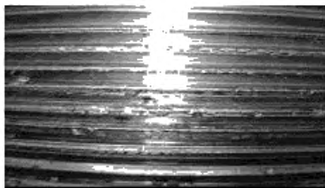
в) Задир на наружной резьбе после свинчивания
