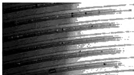
а) Задирь на внутренней резьбе после нарезания резьбы
