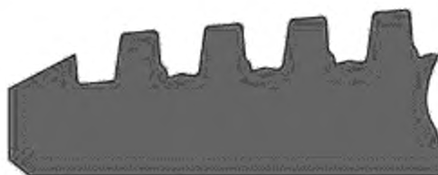
б) Уступы во впадинах витков трапецидальной резьбы
