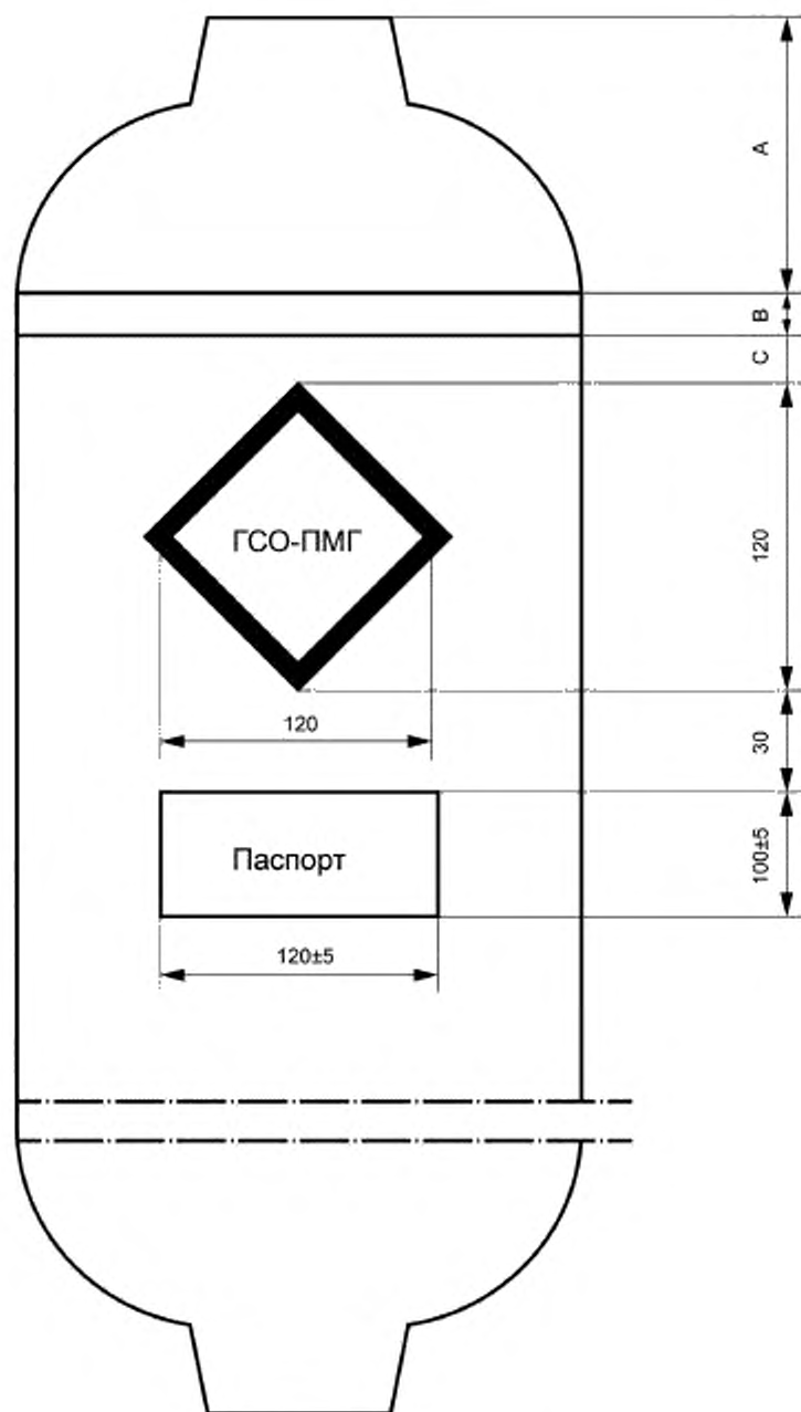
Рисунок В.1 — Маркировка баллона
