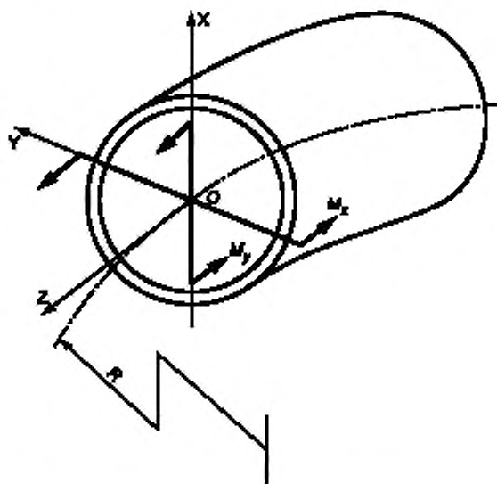
Рисунок 13 — Изгибающие моменты в сечении криволинейной трубы
