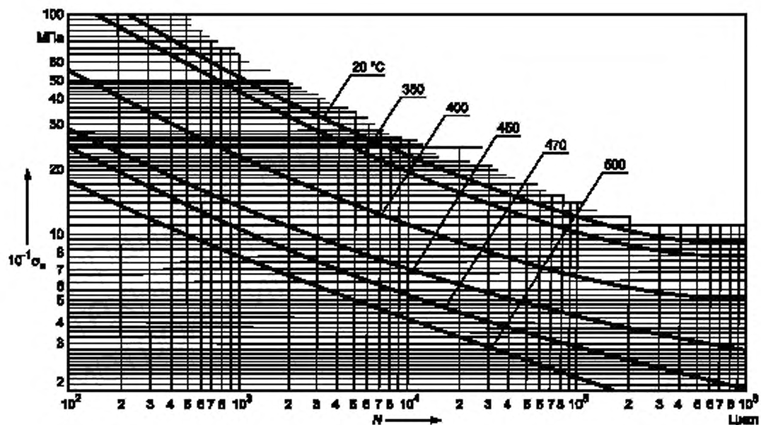
Рисунок 2 — Расчетные кривые малоциклового усталости углеродистых сталей
