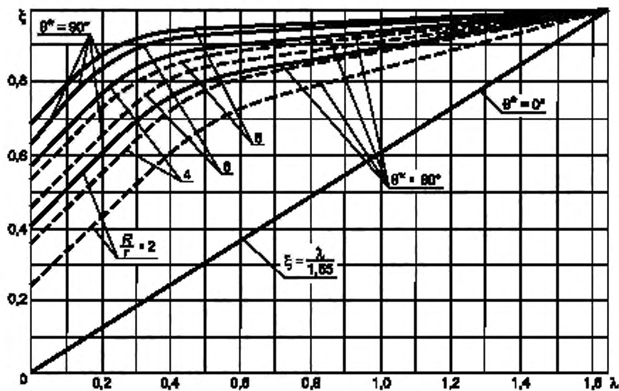
Рисунок 8 — Коэффициент \xi
