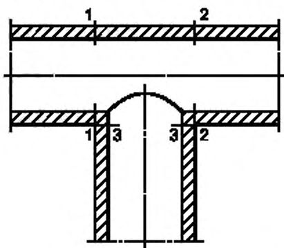
Рисунок 12 — Расчетные сечения тройникового узла
