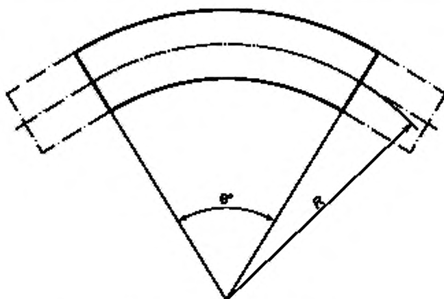
Рисунок 7 — Криволинейная труба
