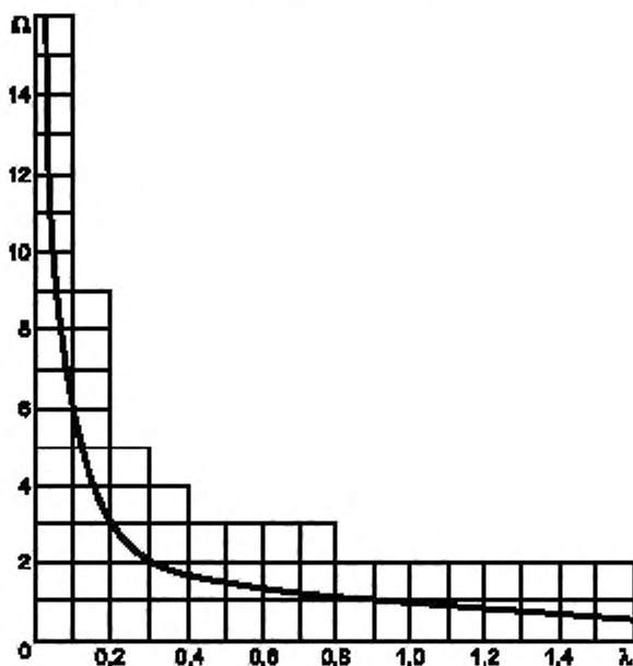
Рисунок 10 — Коэффициент \Omega
