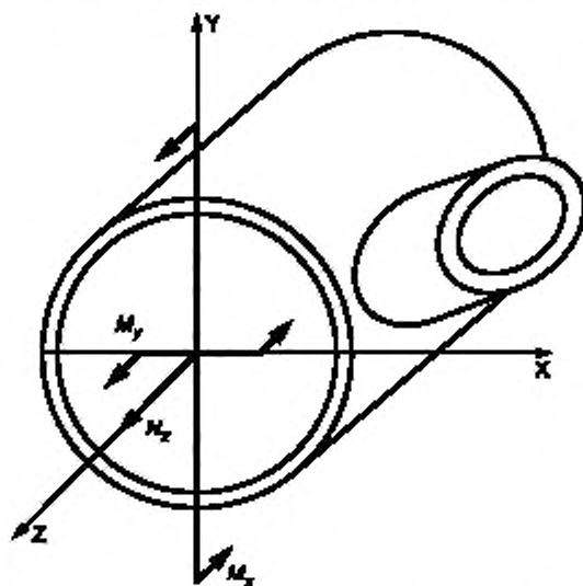
Рисунок 14 — Силовые факторы в поперечном сечении тройникового узла
