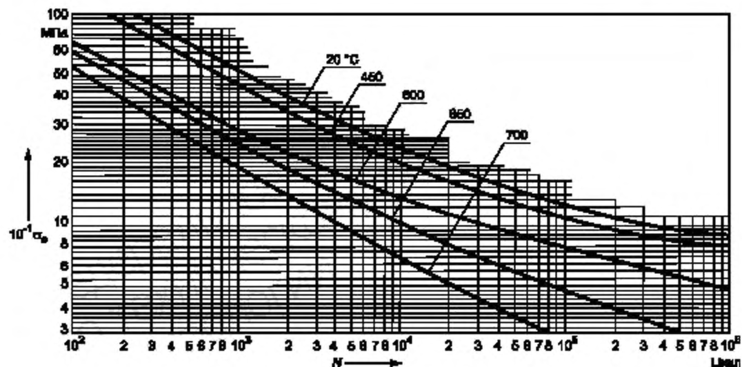
Рисунок 4 — Расчетные кривые малоциклового усталости аустенитных хромоникелевых сталей
