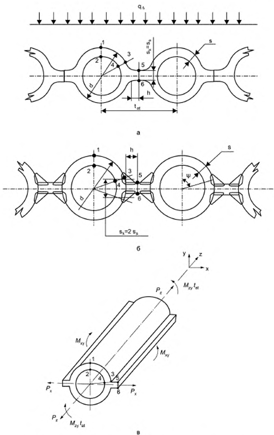
а — мембранный экран из сварных труб; б — мембранный экран из гладких труб; в — схема приложения усилий и моментов к оребренной трубе
