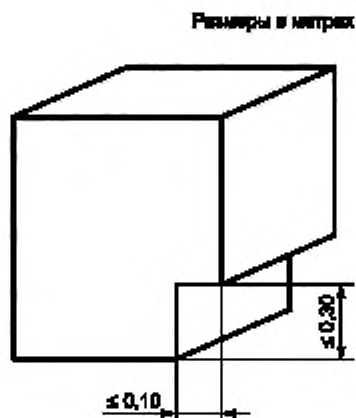
Рисунок 4 — Максимальные уменьшения пространств безопасности для персонала
