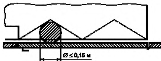
Рисунок 8 — Распашная дверь шахты и складная дверь кабины
