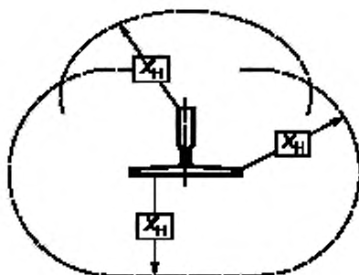
Рисунок 6 — Горизонтальное расстояние X_{H1} вокруг направляющей
