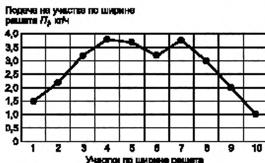
Рисунок Г.1 — График распределения обрабатываемого материала по ширине решета
