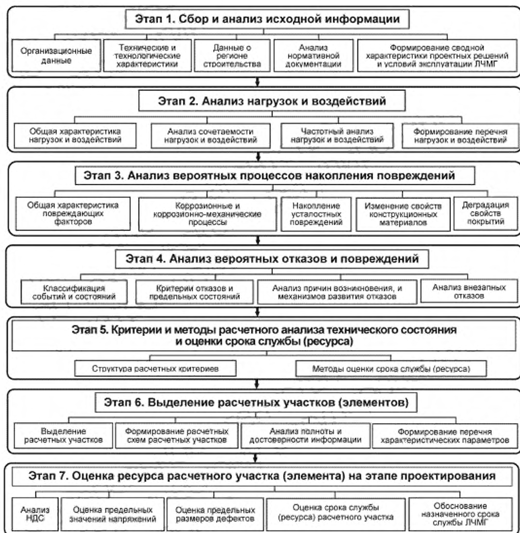
Рисунок А.1 — Схема алгоритма оценки срока службы (ресурса) ЛЧМГ при проектировании
