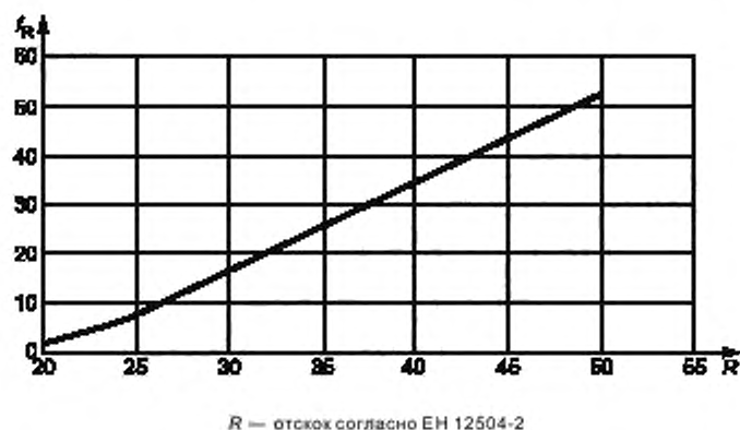
Рисунок 2 — Базовая кривая для испытаний на упругий отскок
