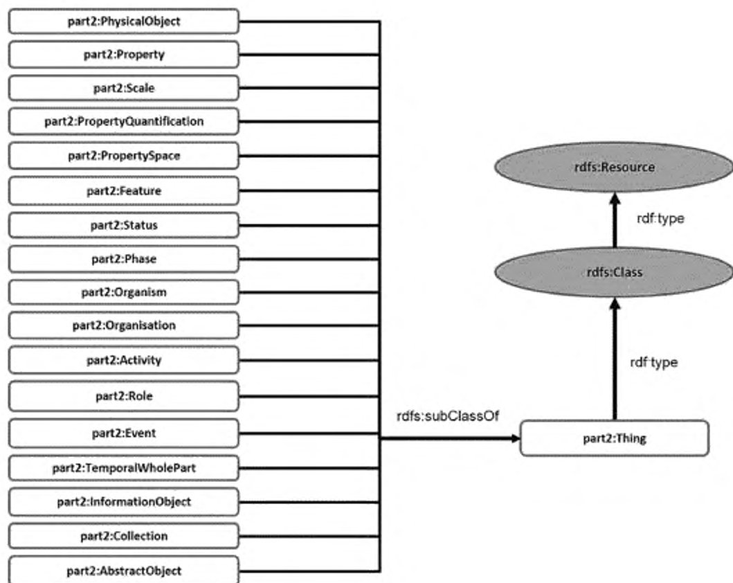
Рисунок 8 — Расширение RDF базовыми классами RDL путем мэппинга rdfs:Class в part2:thing
