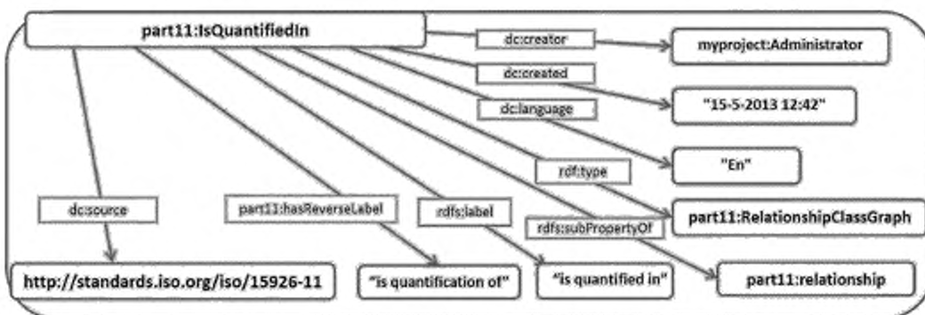
Рисунок 23 — Именованный RDF-граф, представляющий взаимосвязь part11 с меткой (обозначением) «is quantified in»
