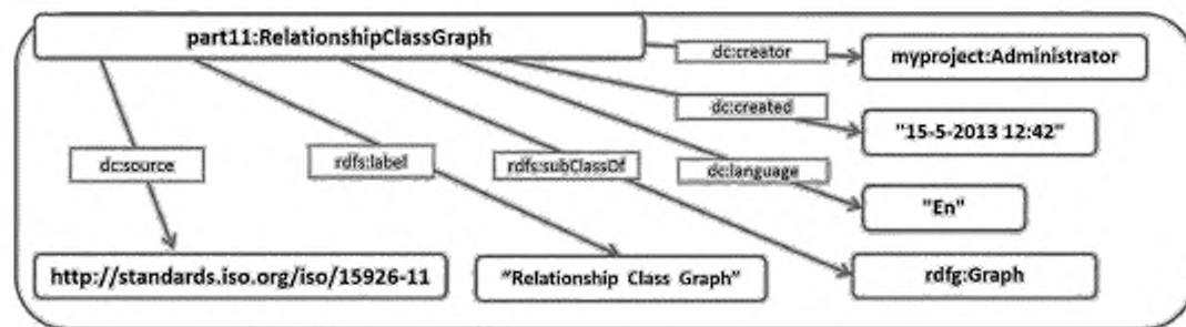
Рисунок 14 — Именованный граф, представляющий класс «RelationshipClassGraph»
