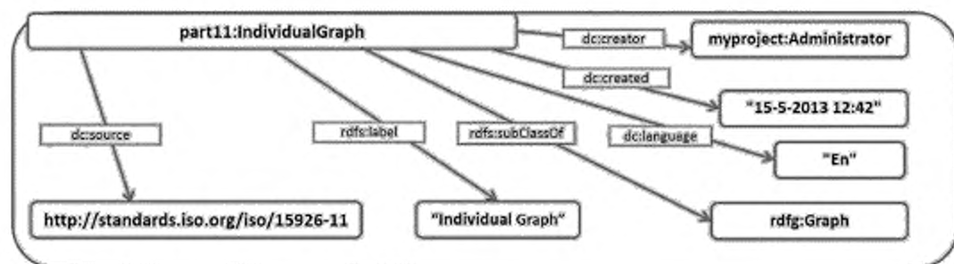
Рисунок 13 — Именованный граф, представляющий класс «part11:IndividualGraph»
