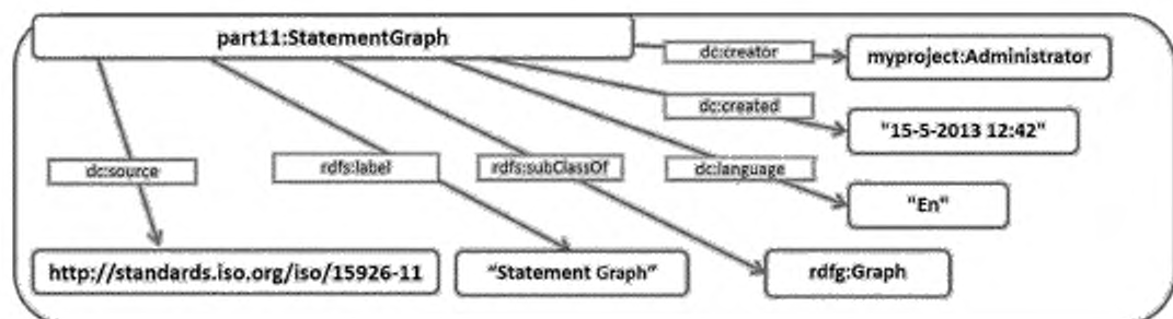
Рисунок 15 — Именованный RDF-граф, представляющий класс «StatementGraph»
