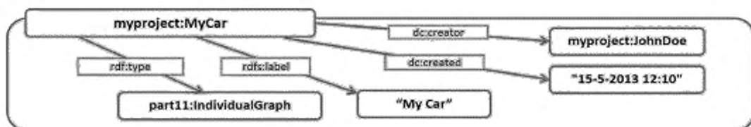
Рисунок 17 — Именованный RDF-граф, представляющий место для заполнения для «MyCar»
