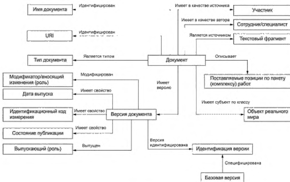
Рисунок 73 — Информационная модель, представляющая информацию о документе
