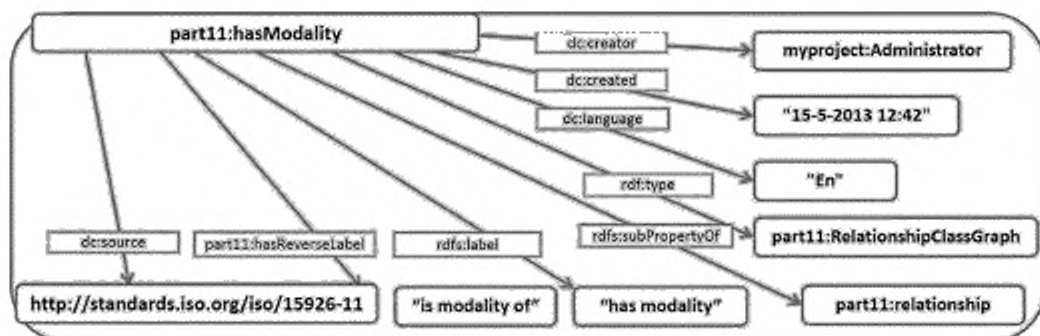
Рисунок 22 — Именованный RDF-граф, представляющий взаимосвязь части 11 с меткой (обозначением) «has modality»
