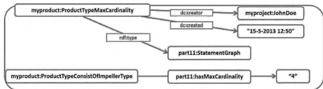
Рисунок 51 — Именованный RDF-граф, указывающий на то, что экземпляр класса myproduct:ProductTypeMaxCardinality состоит, как максимум, из четырех экземпляров myproduct:ImpellerType «4»
