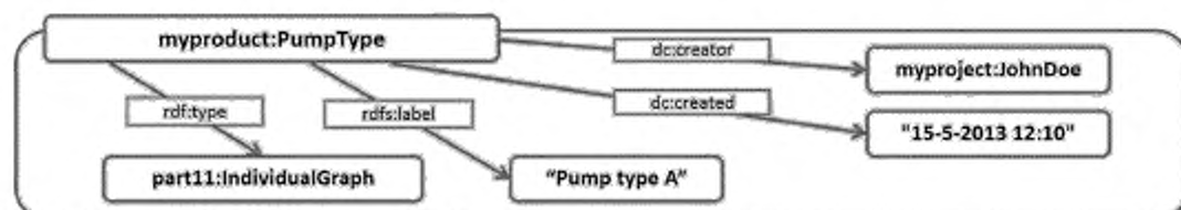
Рисунок 41 — Именованный RDF-граф, представляющий место заполнения для «PumpType» (тип насоса)
