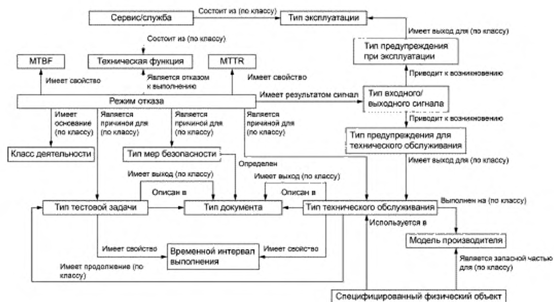
Рисунок 62 — Информационная модель, представляющая режим отказов и анализ воздействий системы путем определения соответствующих элементов и взаимосвязей между этими элементами
