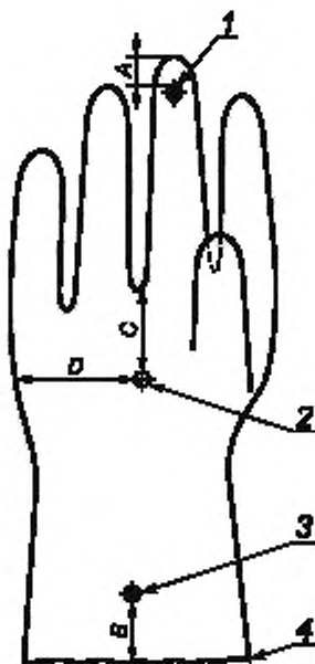
1 — кончик пальца, 2 — ладонь; 3 — манжета; 4 — край манжеты; A = (13 \pm 3) мм; B = (25 \pm 5) мм; C = (33 \pm 7) мм, D = (48 \pm 9) мм (см. примечание 1)
