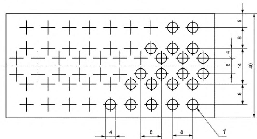
Рисунок А.1 — Конструкция щетки
