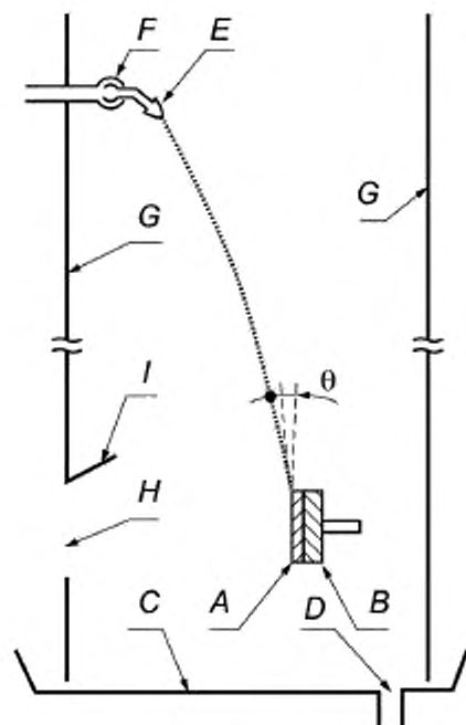
A — проба; B — держатель; C — поддон; D — сточное отверстие; E — струйное сопло; F — шарнирное соединение; G — корпус; H — квадратное отверстие; I — желоб
